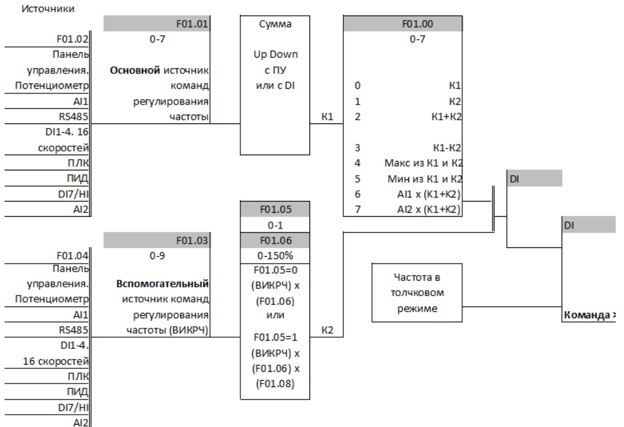
Рис. 6-1 а. Схема выбора источника задания выходной частоты ПЧ
