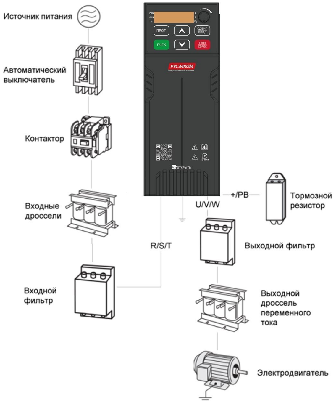
Рис. 3-2. Стандартная конфигурация периферийных устройств
