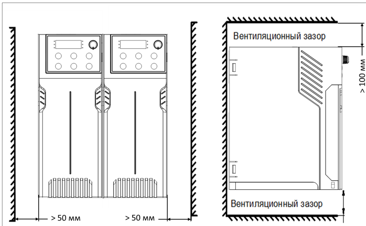
Рис. 3-1. Минимальные расстояния между ПЧ и до стенок шкафа
