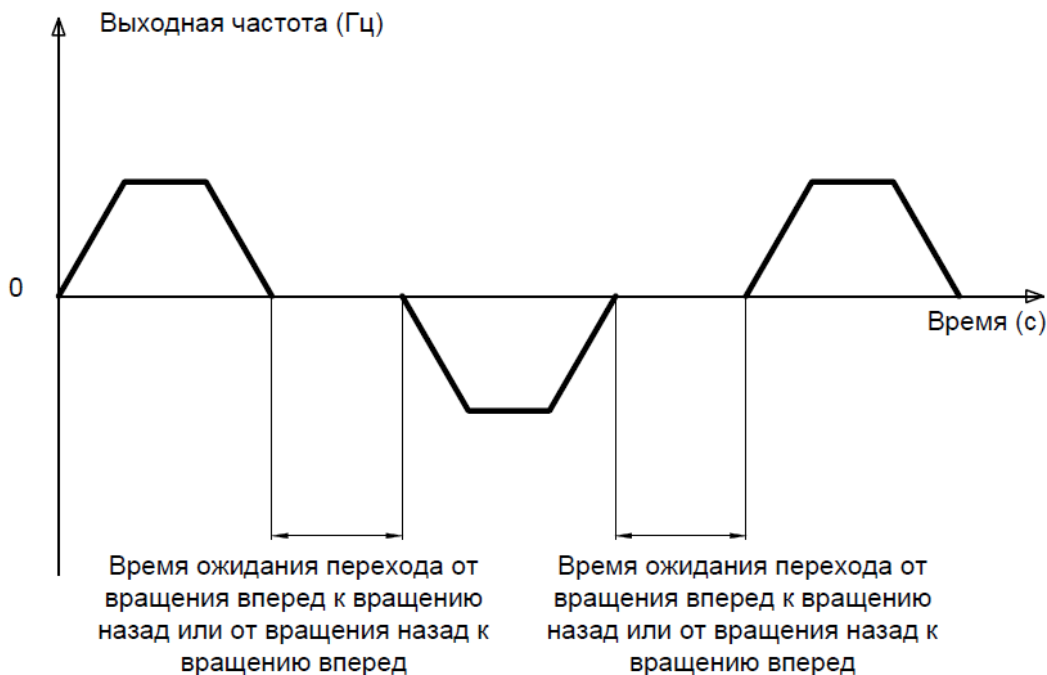
Рис. 6-4. Работа параметра F02.03
