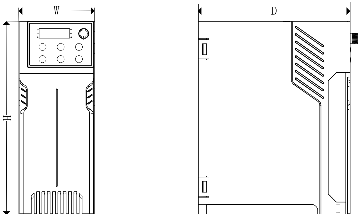
Рис 2-3. Габаритные размеры преобразователей мощностью 0,4 – 7,5 кВт
